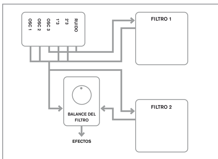
Drum - Como el modo Parallel 2, pero la salida del Filtro 1 es agregada a las señales de entrada del Filtro 2.
