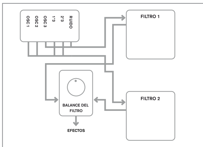
Parallel 2 - Como el modo Parallel, pero el filtro 1 es impulsado por Osc 3 y la fuente de ruido, las fuentes restantes alimentan al filtro 2.
