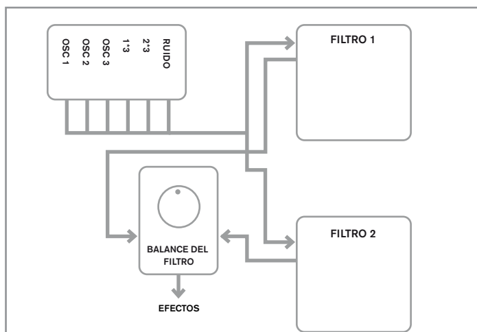
Parallel - Las secciones de filtros son impulsados con la misma señal de entrada, y su mezcla de salida es ajustada con el parámetro Balance del filtro (Filter Balance).
